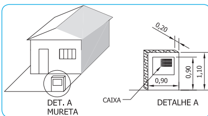
Figura 3 – Instalação em mureta
