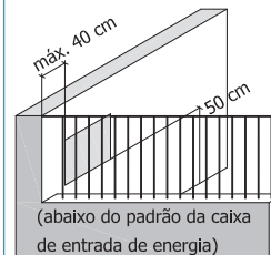
Figura 2 – Instalação em muro lateral
